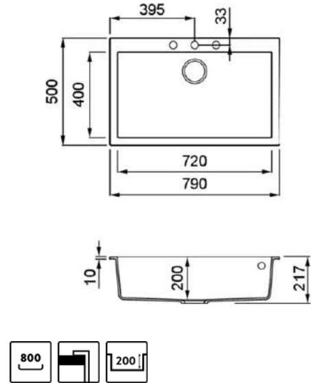
Disegno tecnico
